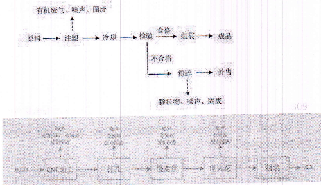
图1 注塑生产工艺及模具生产工艺流程图
